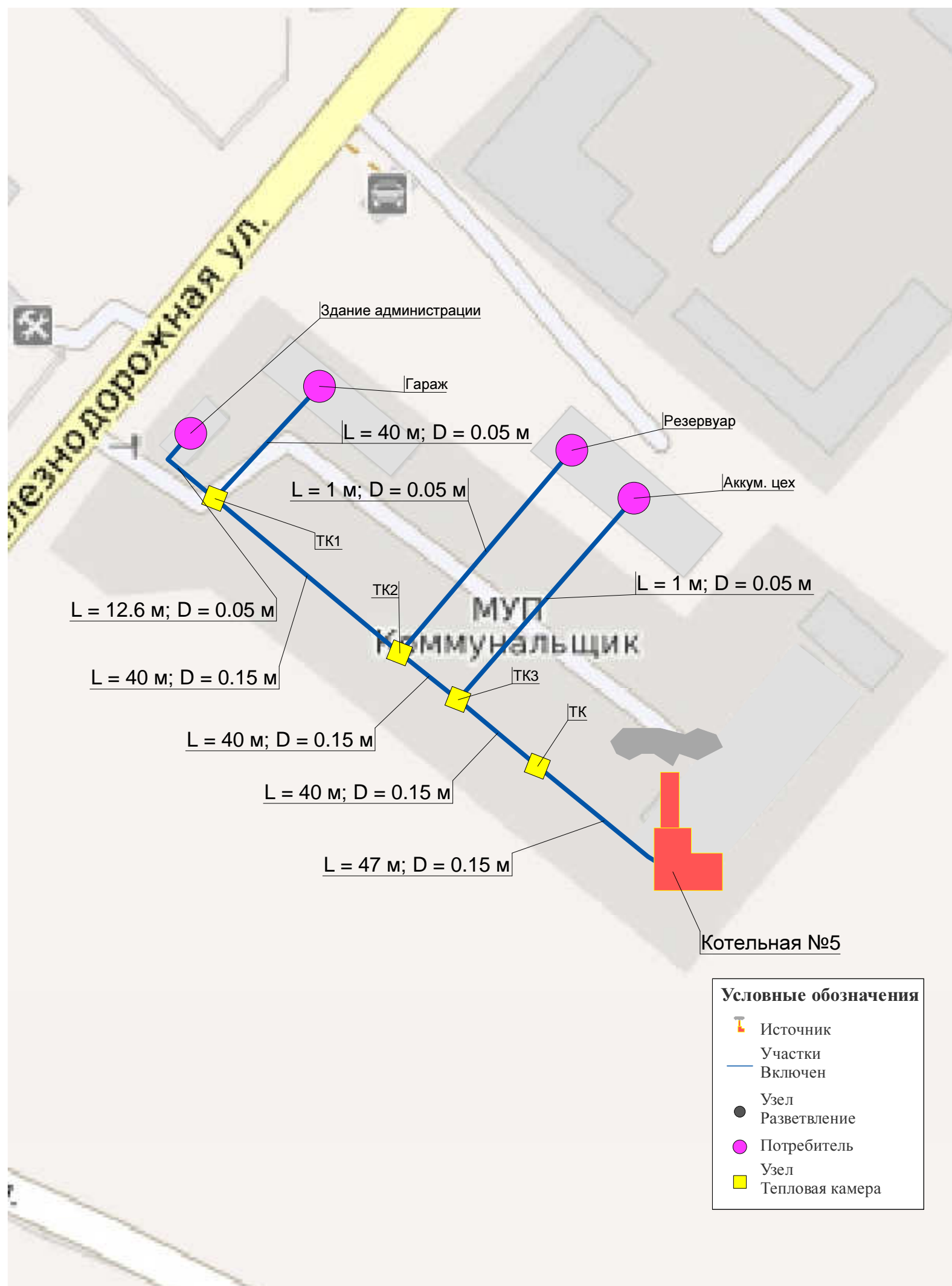
Рис. 3. Схема тепловых сетей п. Ванино Котельной №5
