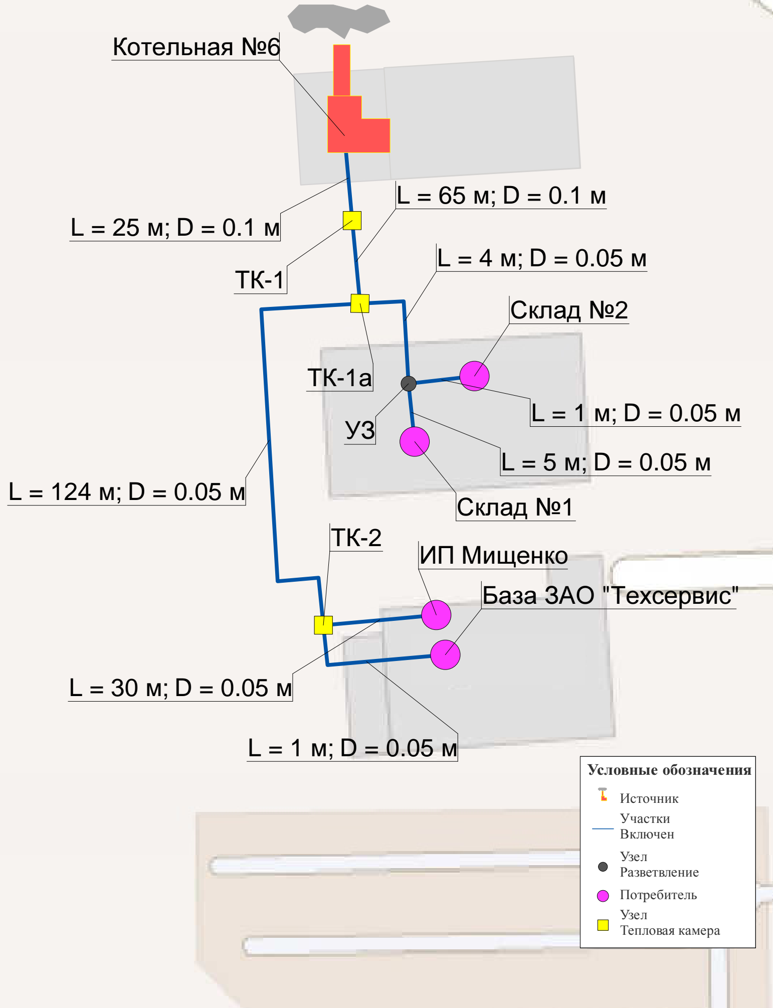
Рис. 4. Схема тепловых сетей п. Ванино Котельной №6
